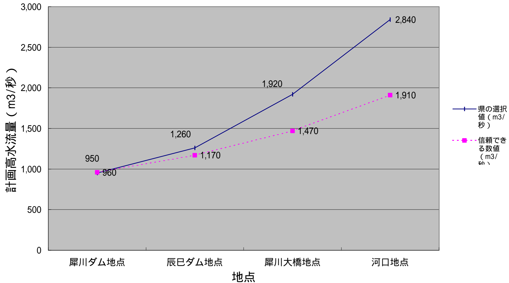
図 計画高水流量（県の選択値と信頼できるデータによる数値との比較）
