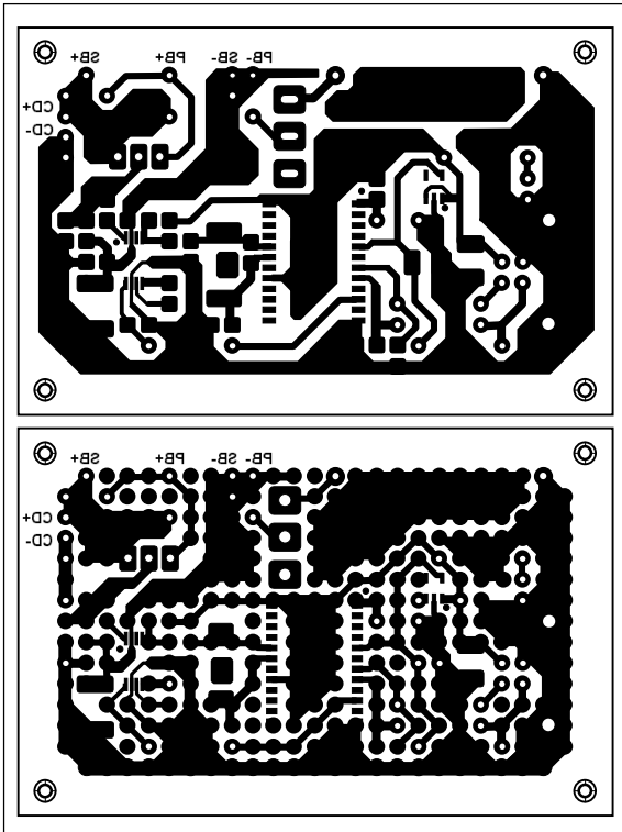
基板サイズ : 71.5 x 46.6 mm Rev.2
